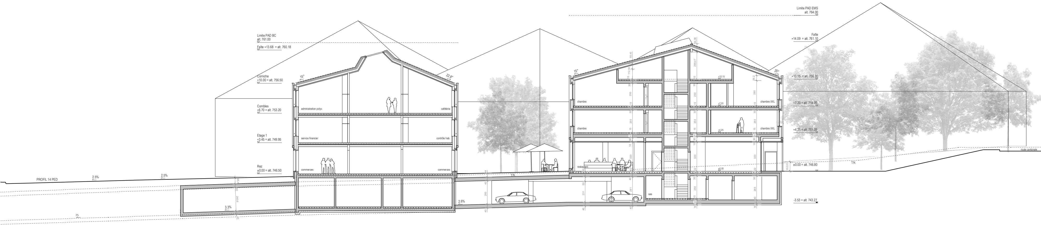
Coupe A-A
